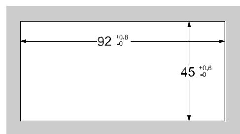
Schalttafelabschnitt gemäß DIN 43700-96x48
