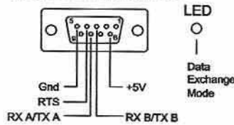
9pol. Sub-D Buchsenleiste
