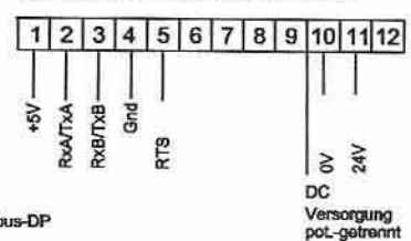
Steckbare Schraubklemmenleiste
