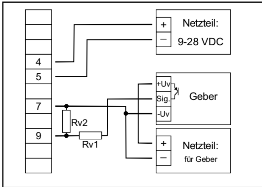
Anschluß eines Gebers (mit getr. Versorgung) mit PNP-Ausgang und externer Widerstandsbeschaltung
